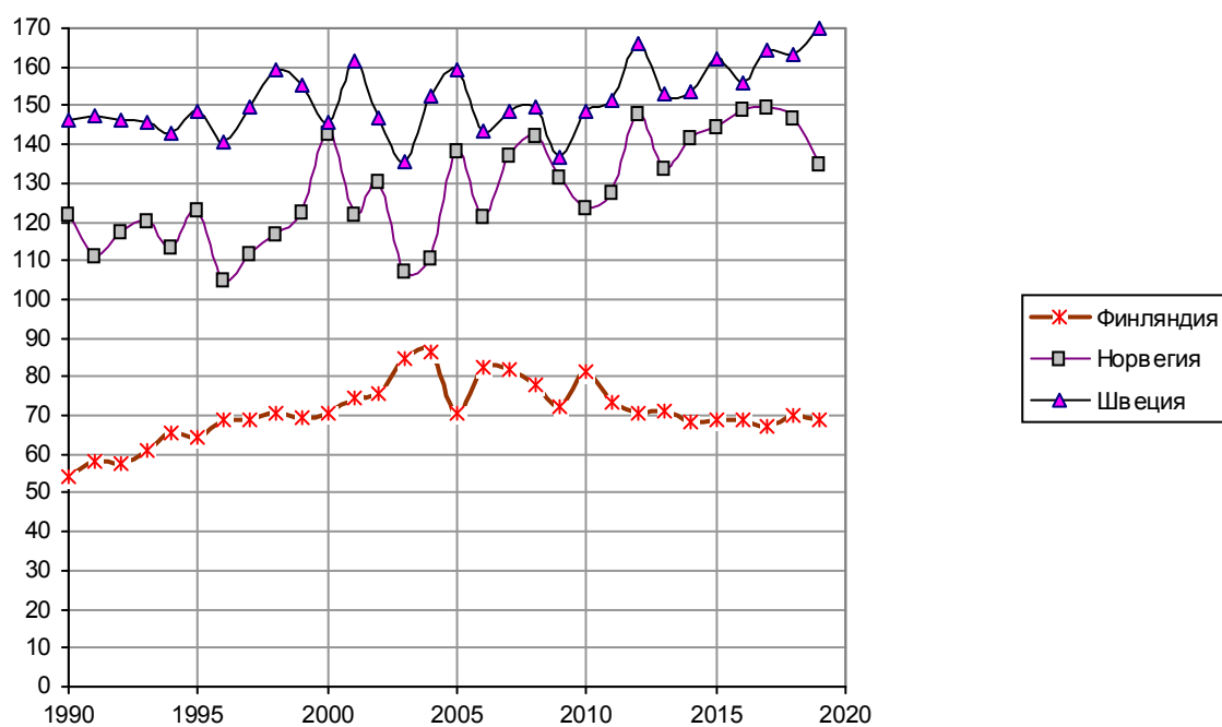
Производство электроэнергии в Финляндии, Норвегии и Швеции, млрд. кВт*ч. Источник: BP Statistical Review of World Energy.
