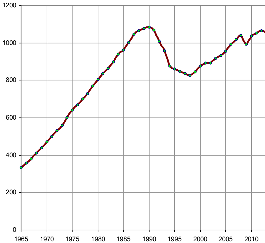
Производство электроэнергии в России, млрд. кВт*ч. Источник: Росстат [1.6].
