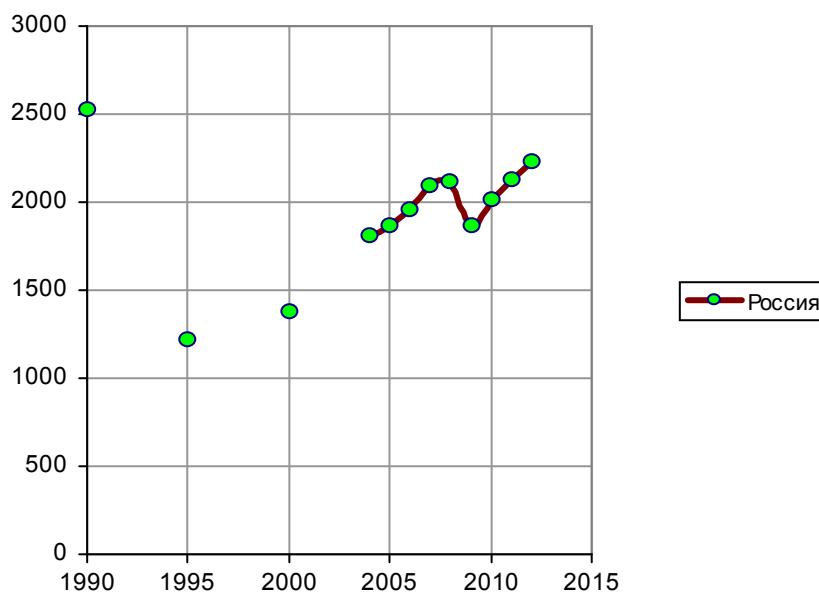
Грузооборот железнодорожного транспорта России, млрд. т-км. Источник: [I.6]
