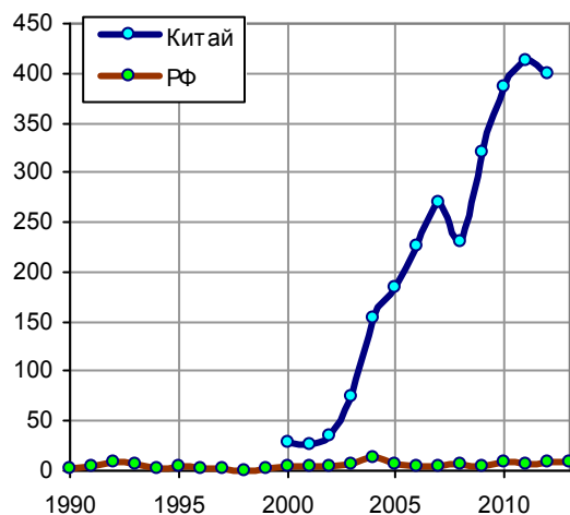
Рис. 1.97, в. Ввод мощностей по добыче угля, млн. т. Источники: [1.6, 1.7]; National Bureau of Statistics of China.
