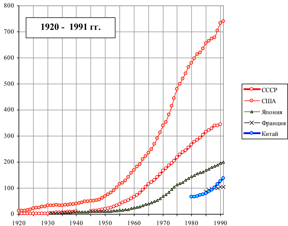
Рис. 1.124, а. Установленная мощность электростанций, млн. кВт. Источники: [1.4, 1.6]; National Bureau of Statistics of China; Japan Statistical Yearbook; U.S. Energy Information Administration (EIA), International Energy; U.S. Census Bureau, Statistical Abstract.
