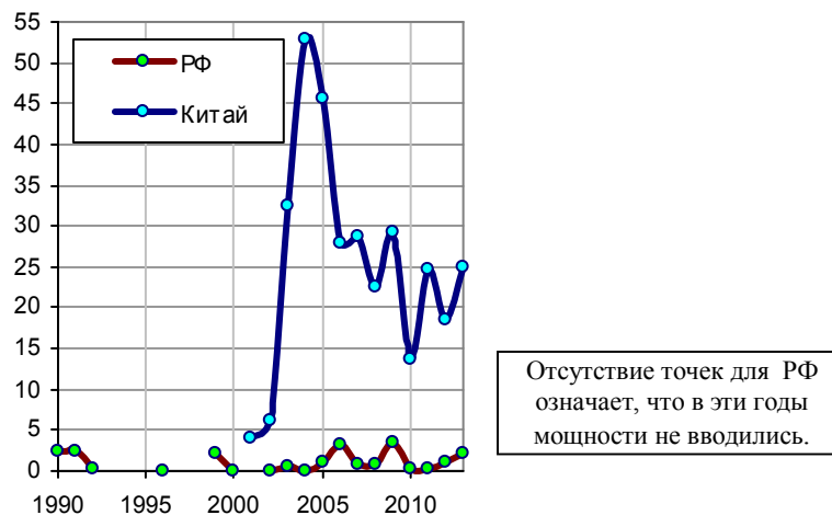
Рис. 1.110. Ввод новых мощностей по выплавке стали, млн. т. Источники: [I.6, I.7]; National Bureau of Statistics of China.
