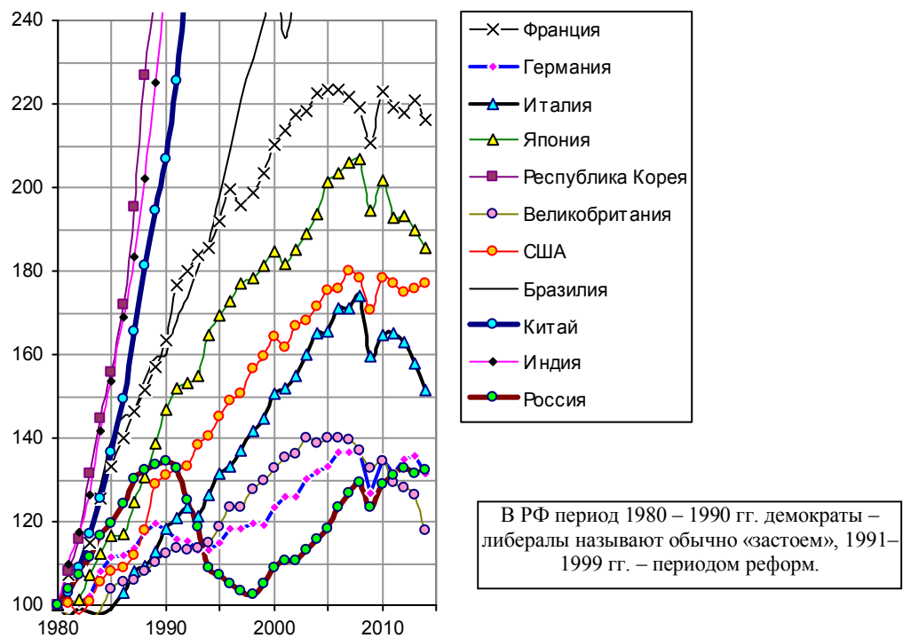
Рис. 1.123. Производство электроэнергии в некоторых странах, 1980 г. – 100. Источники: Electricity Information Administration, EIA; OECD; Japan Statistical Yearbook; BP Statistical Review of World Energy.
